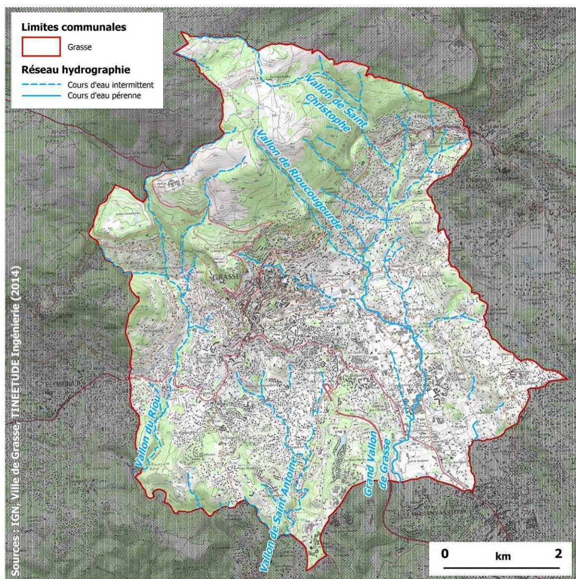
Fig. 4 //Réseau hydrographique (IGN Scan25)
