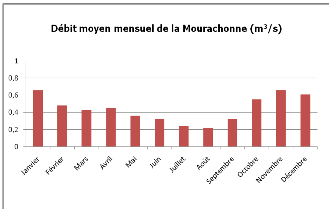
Fig. 118 // Débits moyens mensuels de la Mourachonne à Pégomas (Source : Banque Hydro)
