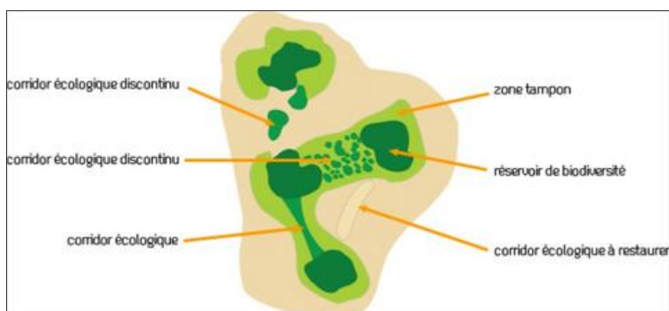
Les continuités écologiques d'après DREAL Provence Alpes-Côtes d'Azur
