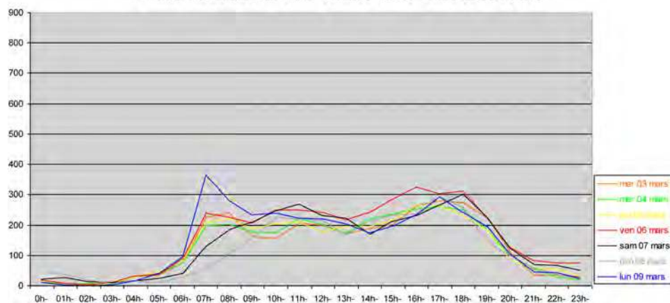
Evolutions horaires de trafic - Avenue Thiers - Sens sortie de ville
