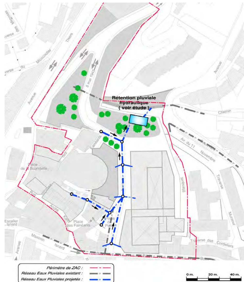
Le réseau des eaux pluviales projeté de collecte du quartier Martelly
