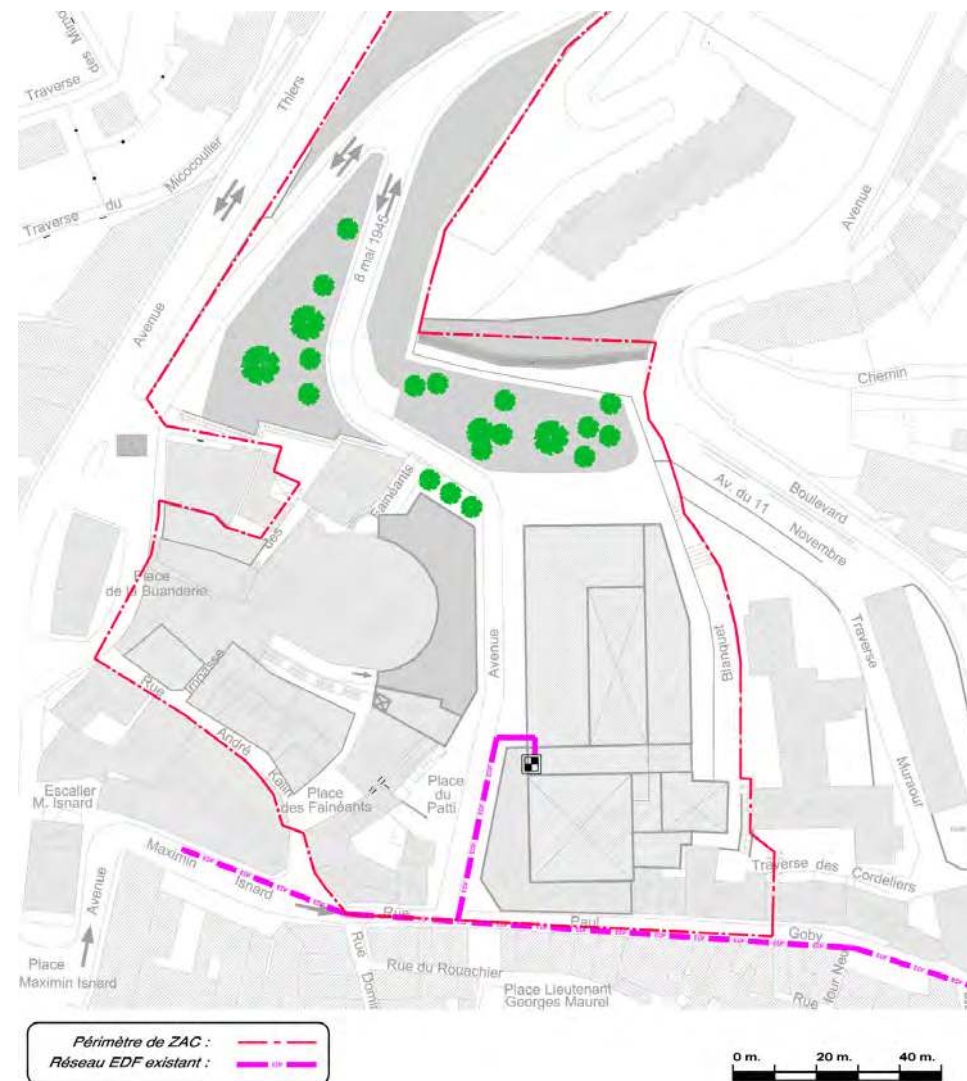
Le réseau d'électricité existant du quartier Martelly
