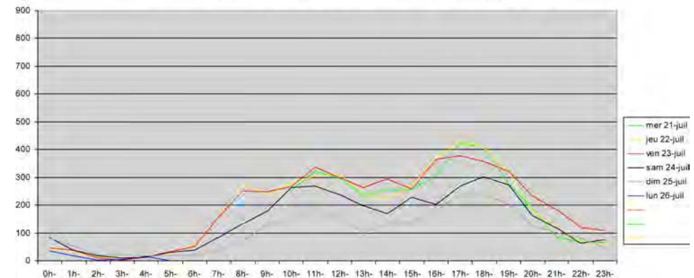
Evolutions horaires des trafics - Avenue Riou Blanquet - Sens Entrée de ville
