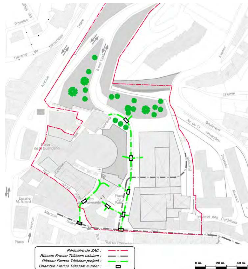
Le réseau projeté de télécommunication du quartier Martelly
