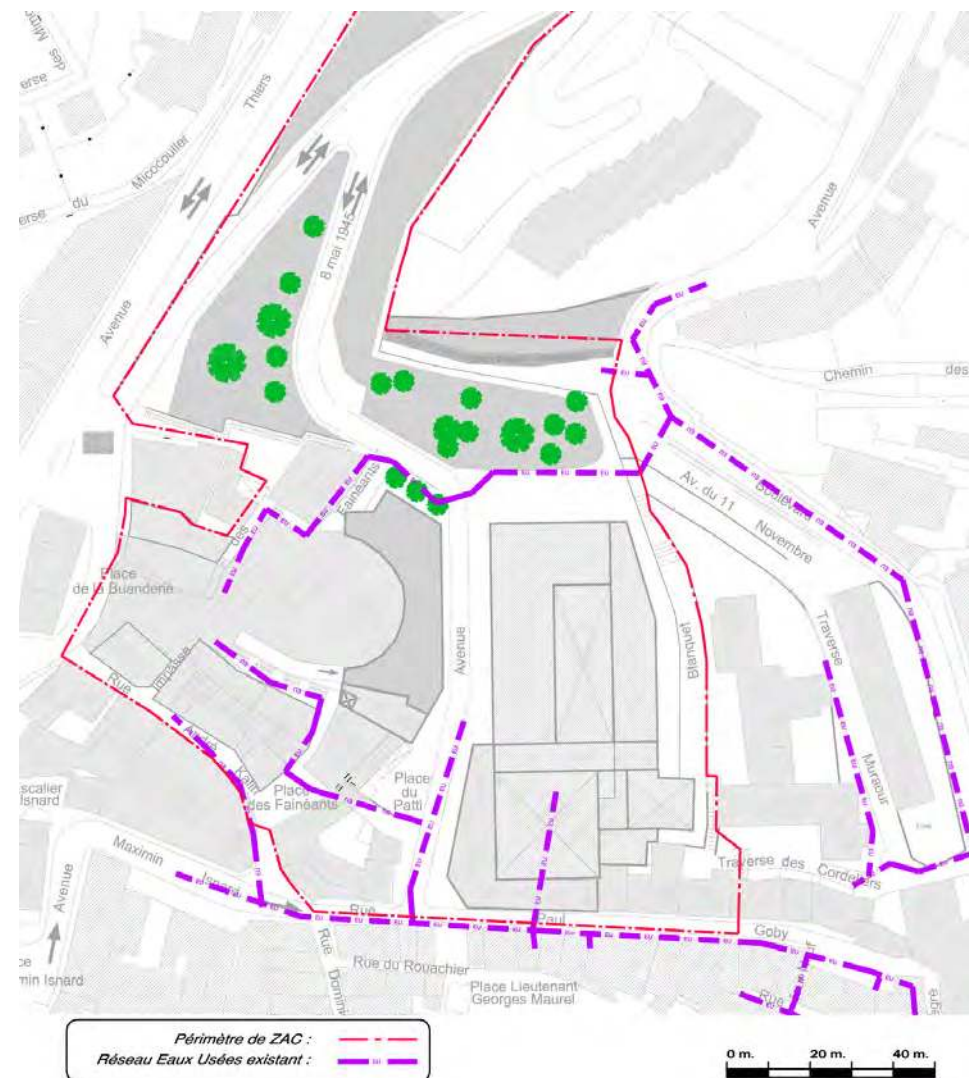
Le réseau d'assainissement existant du quartier Martelly
