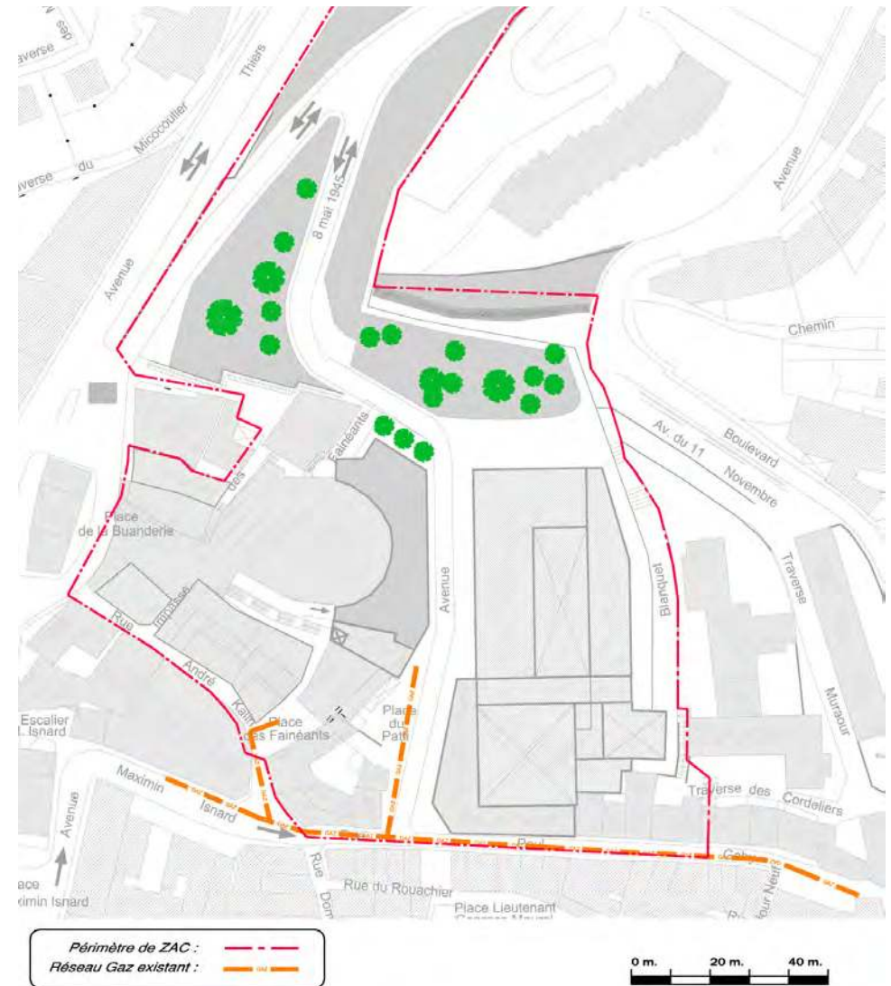
Le réseau de gaz existant du quartier Martelly
