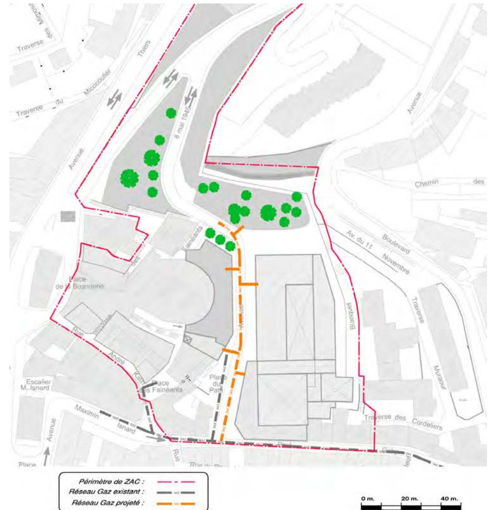
Le réseau projeté de Gaz du quartier Martelly
