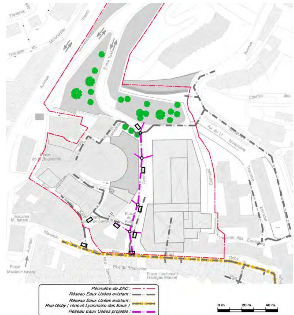
Le réseau projeté d'assainissement collectif du quartier Martelly
